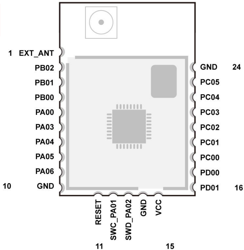
图 3. 引脚图
