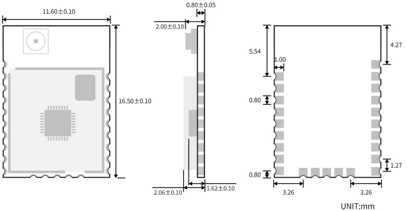
图 2. 尺寸图
