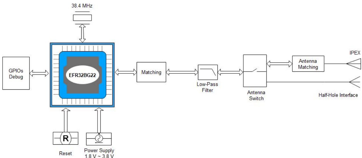
图 1. 原理框图
