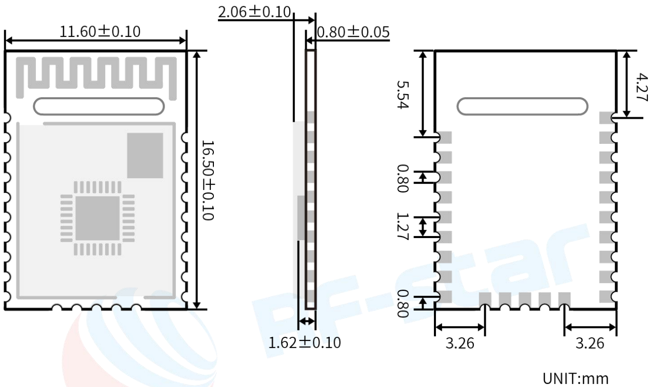
RF-BM-BG22A1/A2/A3 尺寸图
