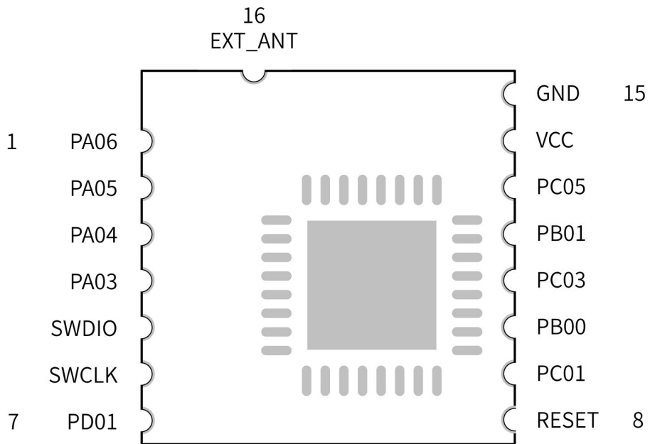
引脚定义图
